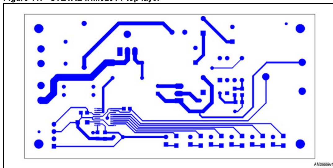
Figure 11. STEVAL-IHM029V1 top layer
