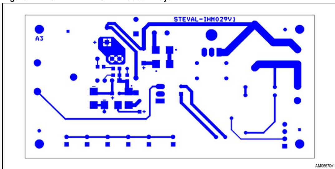
Figure 12. STEVAL-IHM029V1 bottom layer
